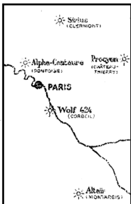
Les 5 plus proches étoiles en 1939
